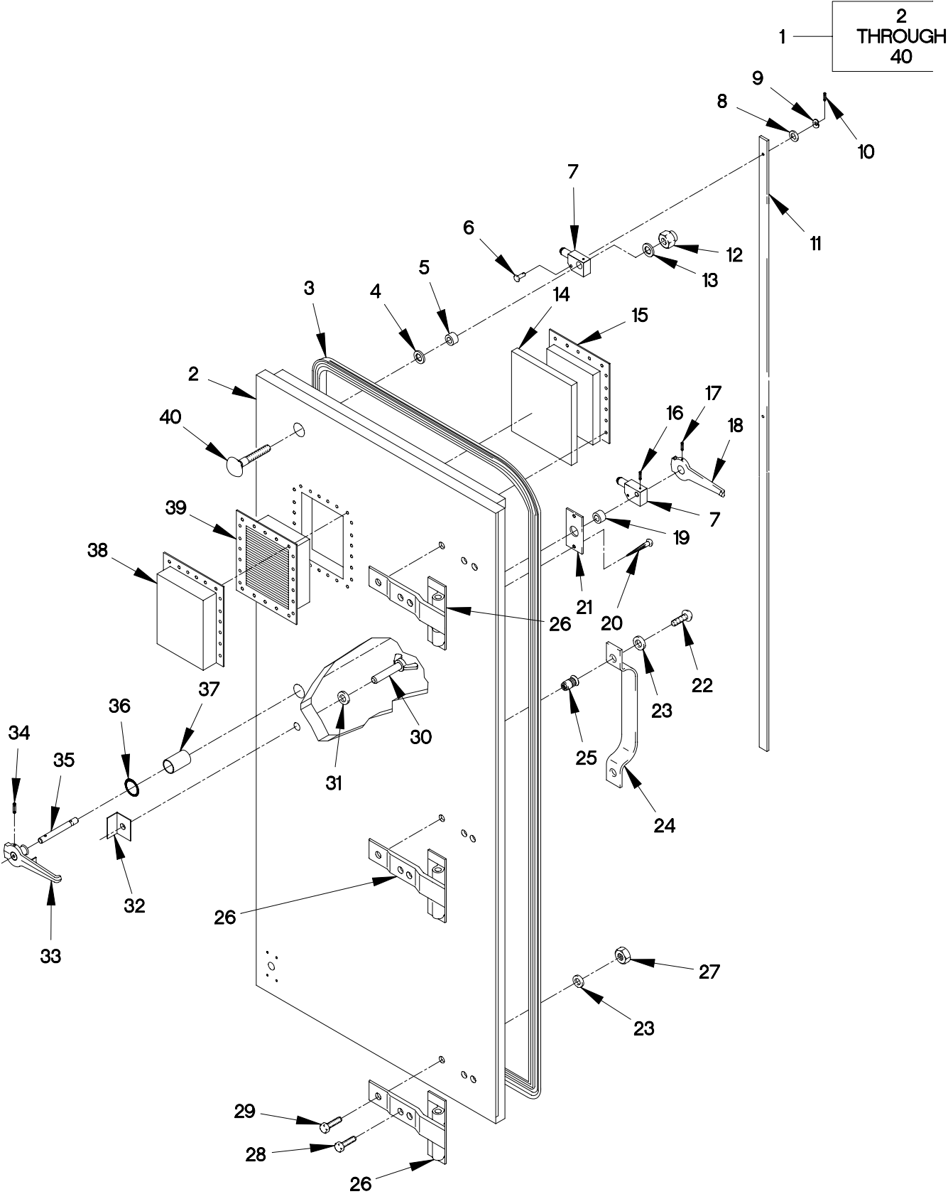
FIGURE 223. VAN RIGHT HAND DOOR (S/N 1-197)
